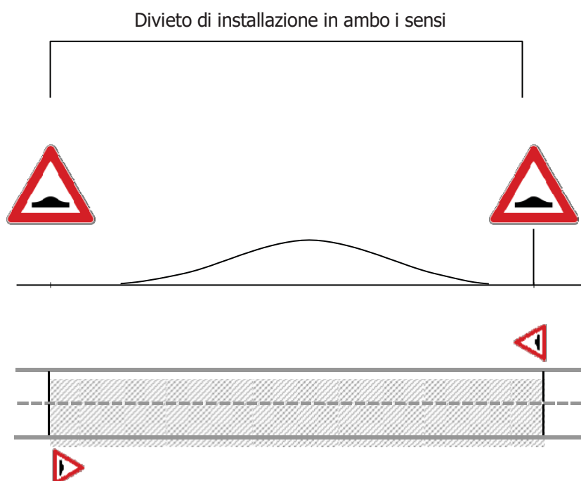
Figura 5. Raccordi verticali concavi e convessi segnalati (dossi e cunette) [Art. 37, comma 2, parte 2.a, lett. g) Reg.]
