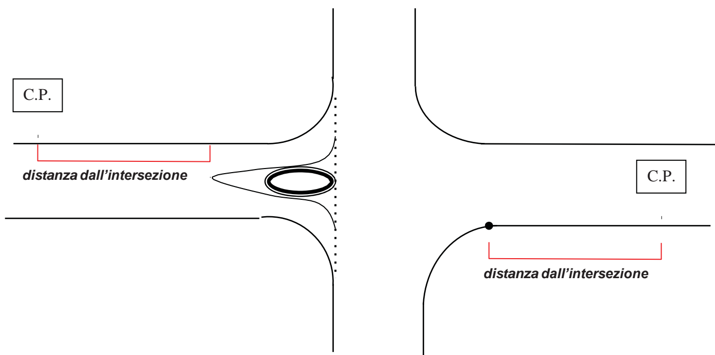
Figura 7.c Distanza dalle intersezioni: intersezione con aiuola spartitraffico [Art. 37, comma 3, lett. c) - Reg.]
