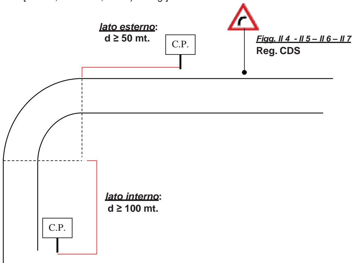
Figura 8.b Distanza dalle curve in presenza della segnaletica di pericolo di cui alle Figg. II 4 - II 5 - II 6 - II 7 [Art. 37, comma 1, lett. e) - Reg.]
