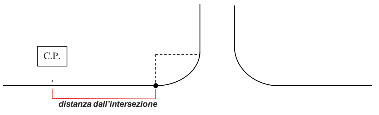
Figura 7.a Distanza dalle intersezioni: intersezione semplice - [Art. 37, comma 3, lett. c) - Reg.]
