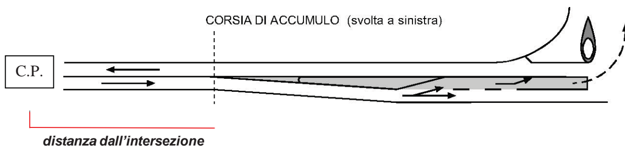
Figura 7.b Distanza dalle intersezioni: intersezione con corsia di accumulo [Art. 37, comma 3, lett. c) - Reg.]
