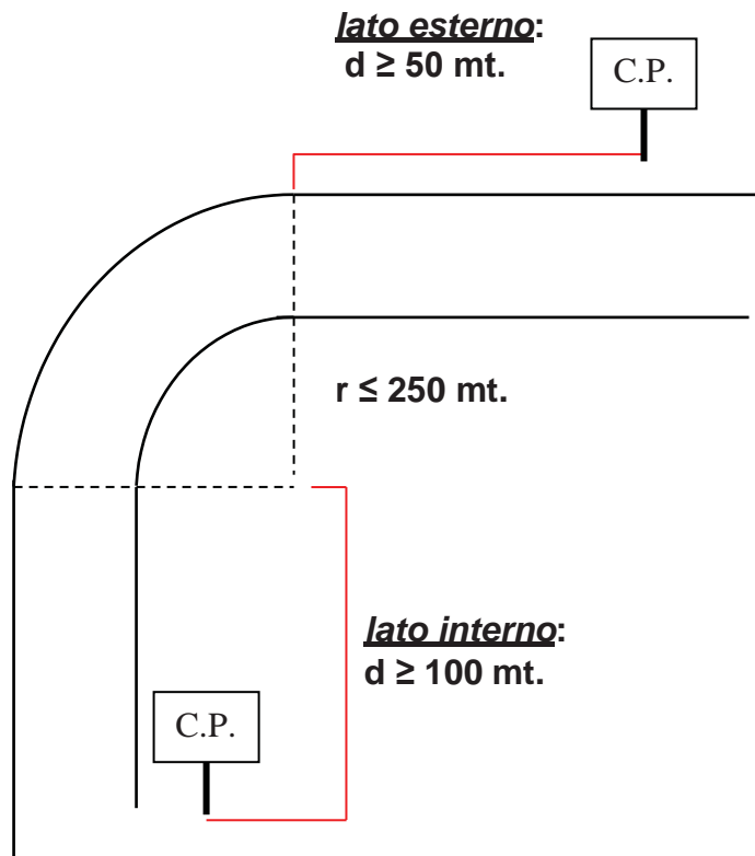
Figura 8.a Distanza dalle curve con raggio inferiore o uguale a 250 mt.- [Art. 37, comma 1, lett. e) - Reg.]
